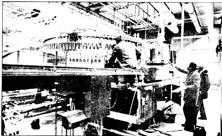
Frá uppsetningu sjálfvirkar átöppunarvélar í nýju sjálfvirkum brugghúsi í Fredericju í Kaupmannahöfn.
